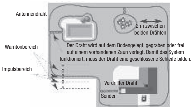
Abb. 3 – Installationsbeispiel
